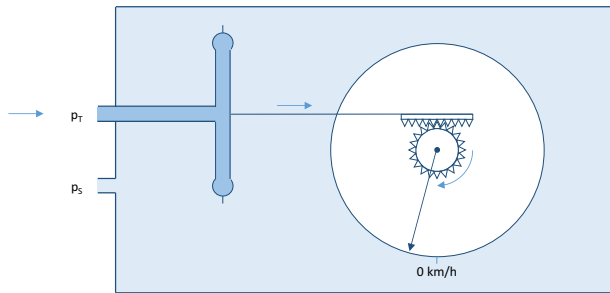
Afbeelding 6-3 Werkingsprincipe snelheidsmeter
