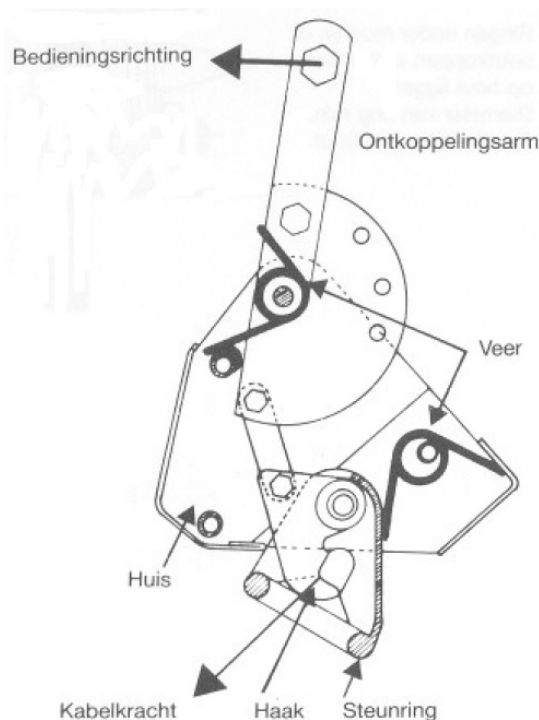
Afbeelding 5-8 Tosthaak
