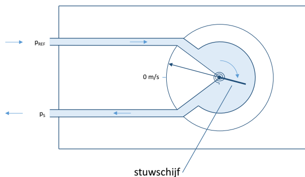
Afbeelding 6-8 Werkingsprincipe stuwschijfvariometer
