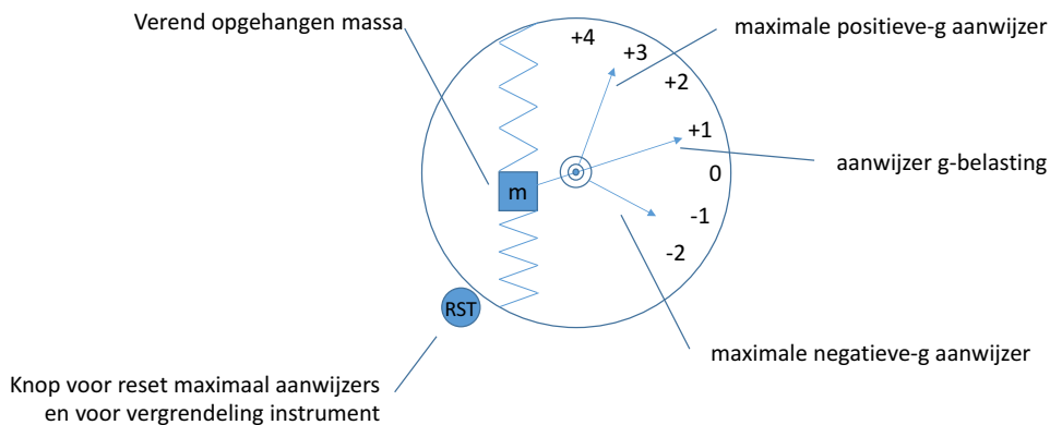
Afbeelding 6-18 g-meter
