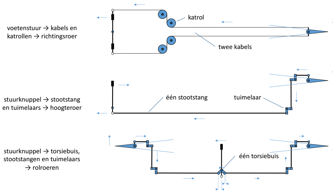
Afbeelding 5-1 Torsiebuis, stootstangen en kabels, katrollen en tuimelaars
