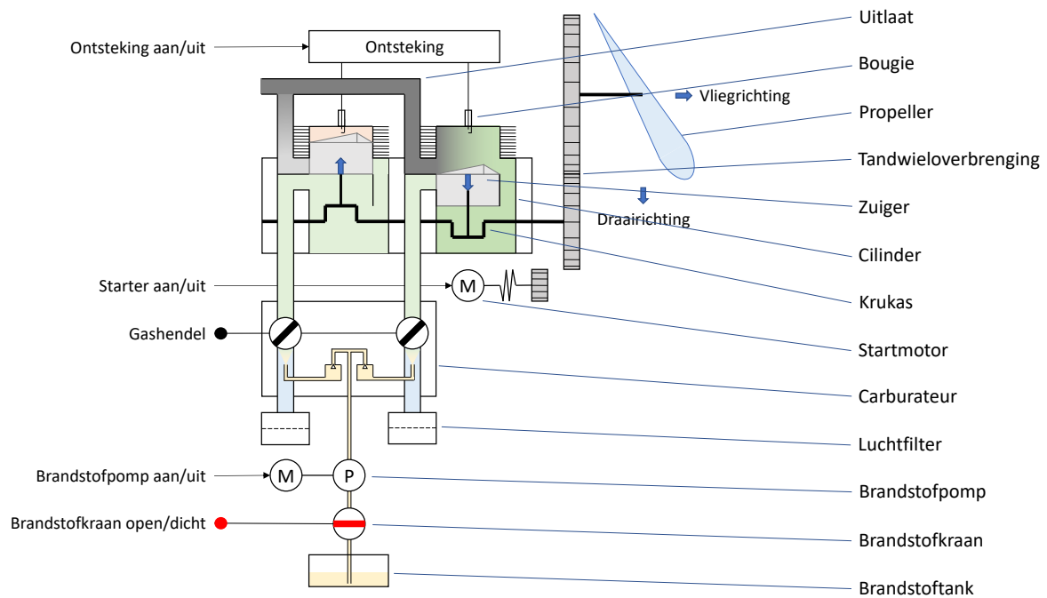
Afbeelding 10-5 Tweecilinder tweetakt-zuigermotor
