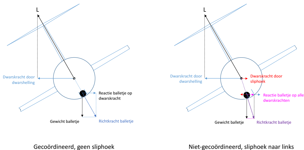
Afbeelding 6-16 Gedrag balletje tijdens vliegen met dwarshelling
