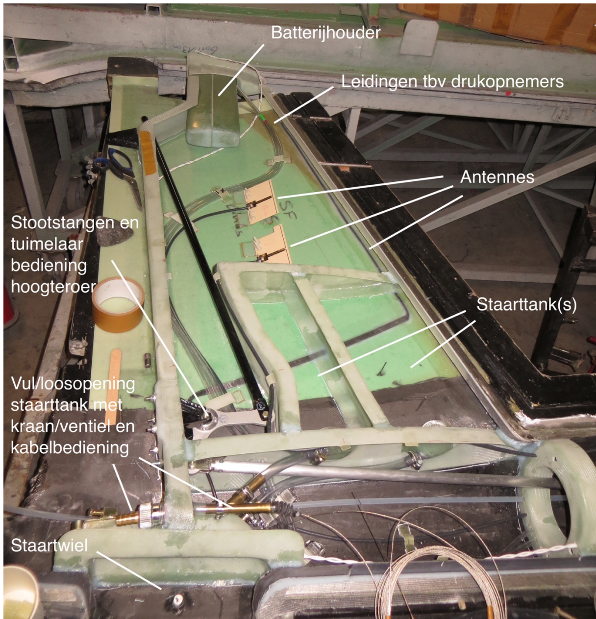
Afbeelding 1-11 Constructie kielvlak (LS10-st)
