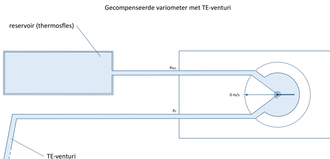
Afbeelding 6-13 Variometer met TE compensatie
