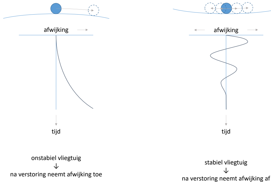
Afbeelding 4-3 Stabiliteit en onstabiliteit
