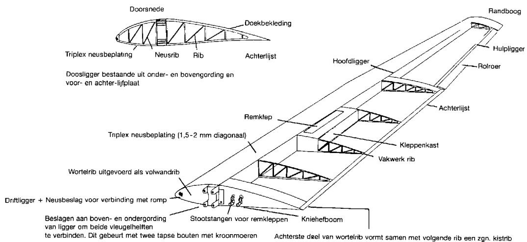
Afbeelding 1-6 Constructie houten vleugel
