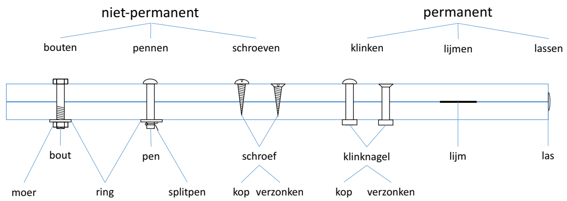
Afbeelding 1-15 Verbindingsmethoden
