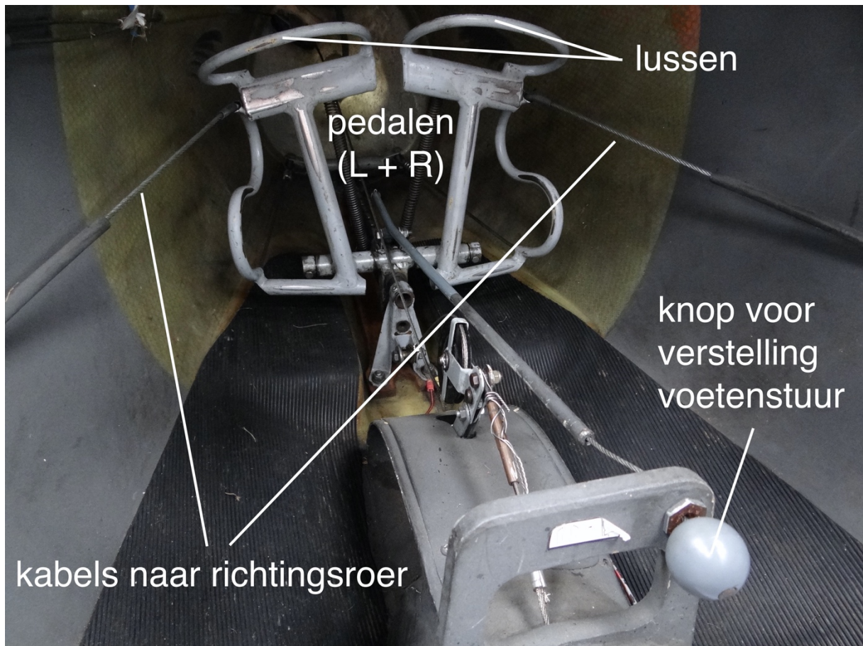
Afbeelding 5-6 Voetenstuur incl. verstelmecanisme (ASK-21)
