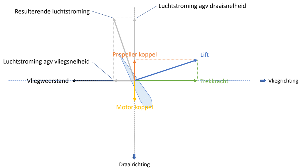
Afbeelding 10-4 Motor-aangedreven propellerblad tijdens de vlucht
