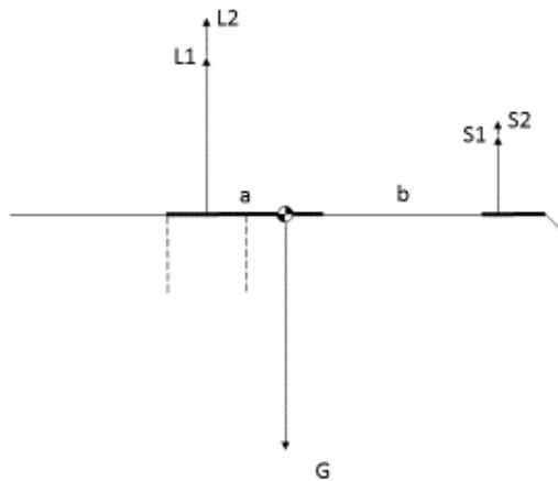
Afbeelding 4-6 Zwaartepunt achter achterste limiet: onstabiel
