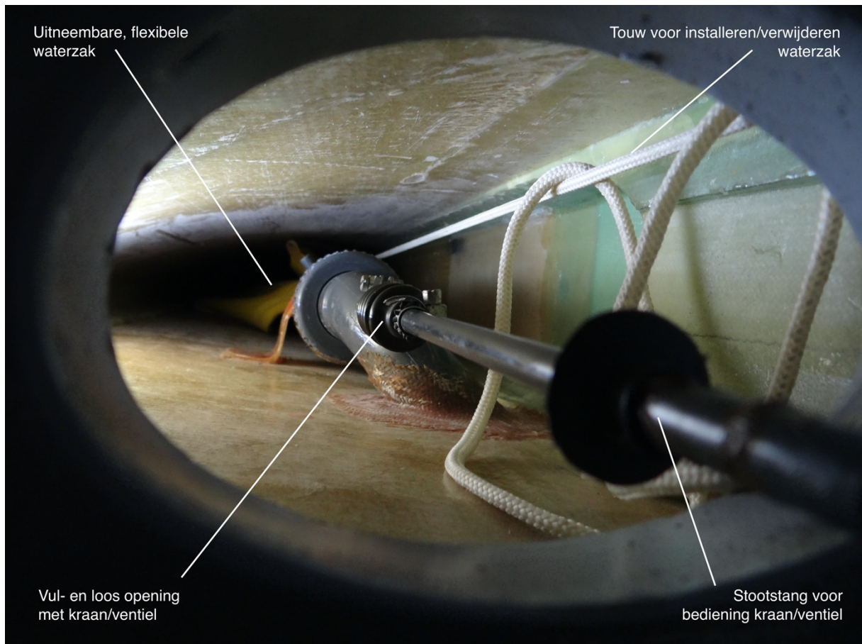
Afbeelding 11-1 Flexibele watertank in vleugelvoorrand (LS4)
