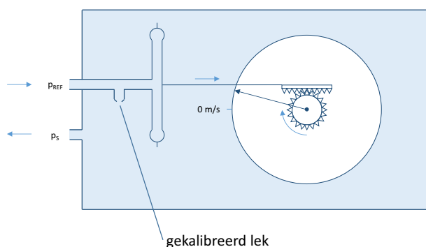
Afbeelding 6-10 Werkingsprincipe variometer met drukcapsule
