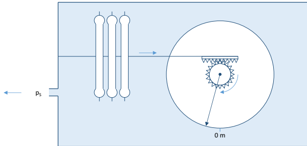
Afbeelding 6-5 Werkingsprincipe hoogtemeter
