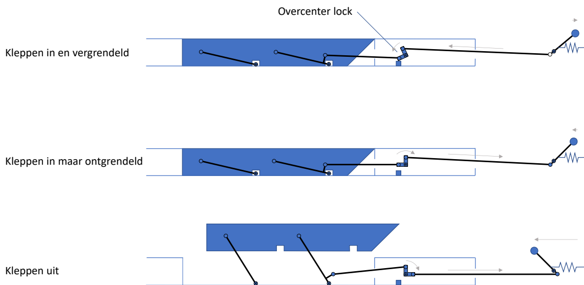
Afbeelding 5-7 Bediening remkleppen
