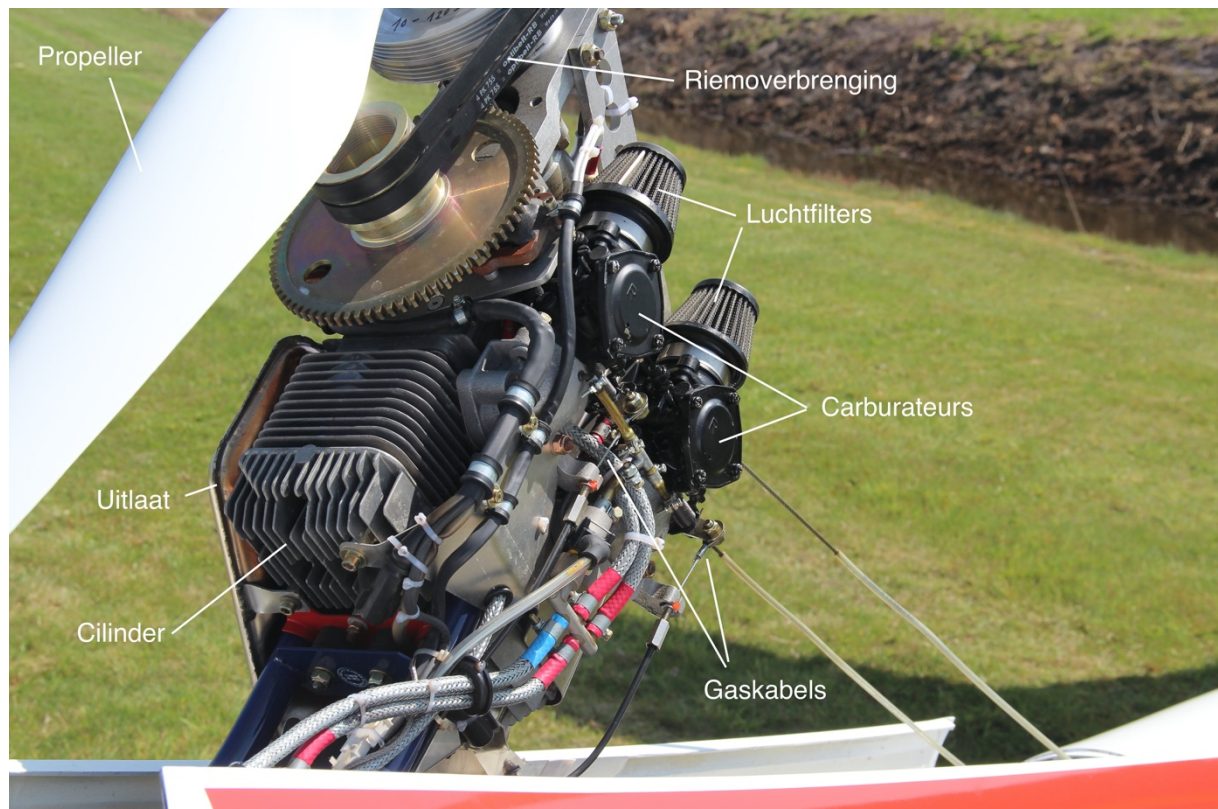
Afbeelding 10-6 Luchtgekoelde twee-cilinder tweetaktmotor met vertragende riemoverbrenging (Solo 2350)
