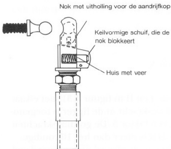
Afbeelding 5-2 l'Hotellier snelkoppeling
