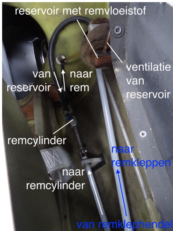
Afbeelding 3-4 Rembediening via klephendel (ASK-21)
