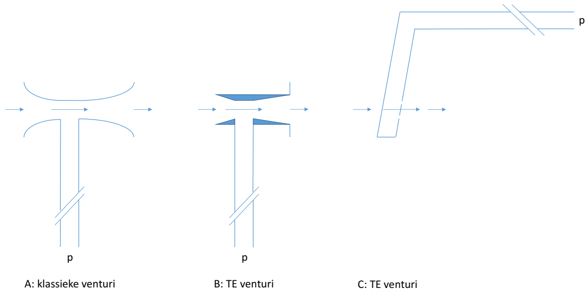
Afbeelding 6-12 TE-venturi buizen
