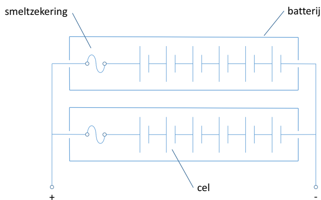
Afbeelding 6-20 Twee parallelle batterijen met elk zes cellen in serie en geïntegreerde smeltzekering
