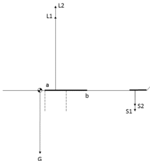
Afbeelding 4-7 Zwaartepunt voor voorste limiet: onbestuurbaar
