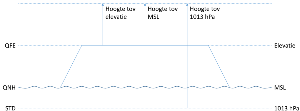
Afbeelding 6-7 Overzicht hoogtemeterinstellingen
