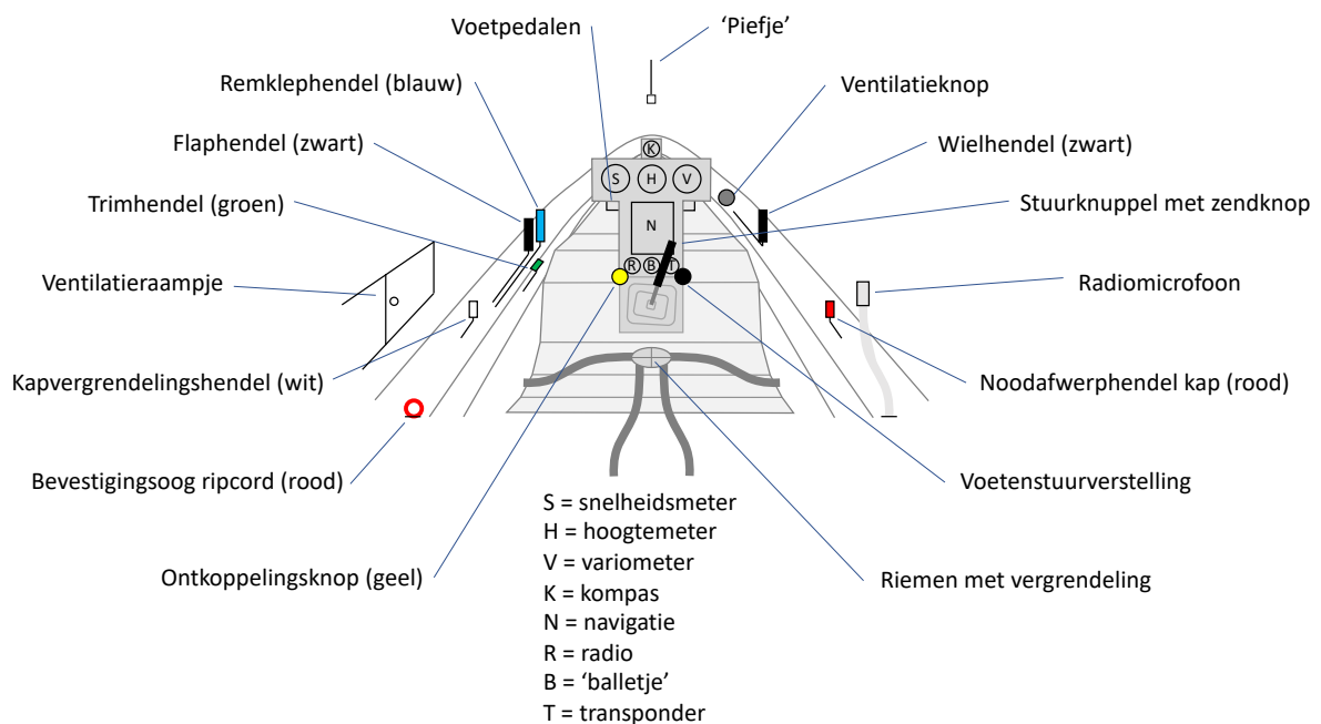
Afbeelding 1-8 Cockpit
