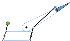
Afbeelding 5-3 Aerodynamische trim en veertrim
