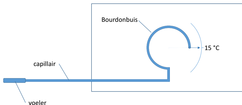
Afbeelding 6-19 Buitenluchttemperatuurmeter
