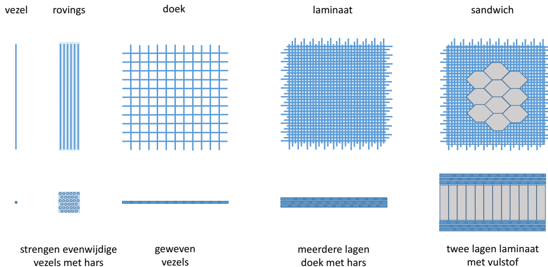
Afbeelding 1-12 Kunststof bouwwijze
