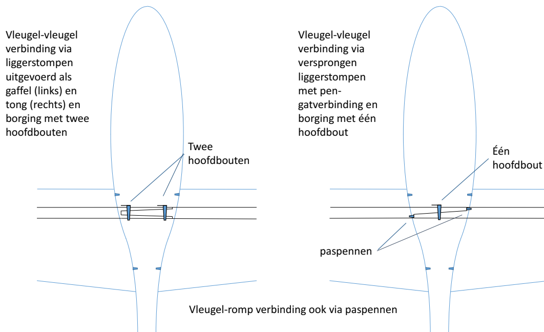
Afbeelding 1-5 In elkaar grijpende vleugelliggers met hoofdbout(en)
