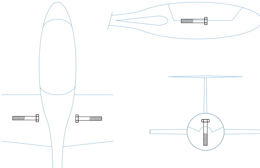
Afbeelding 1-14 Boutbevestigingen
