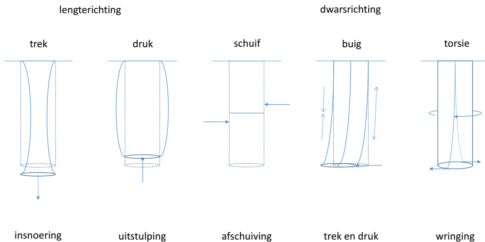
Afbeelding 2-2 Spanningen in lengte- en dwarsrichting
