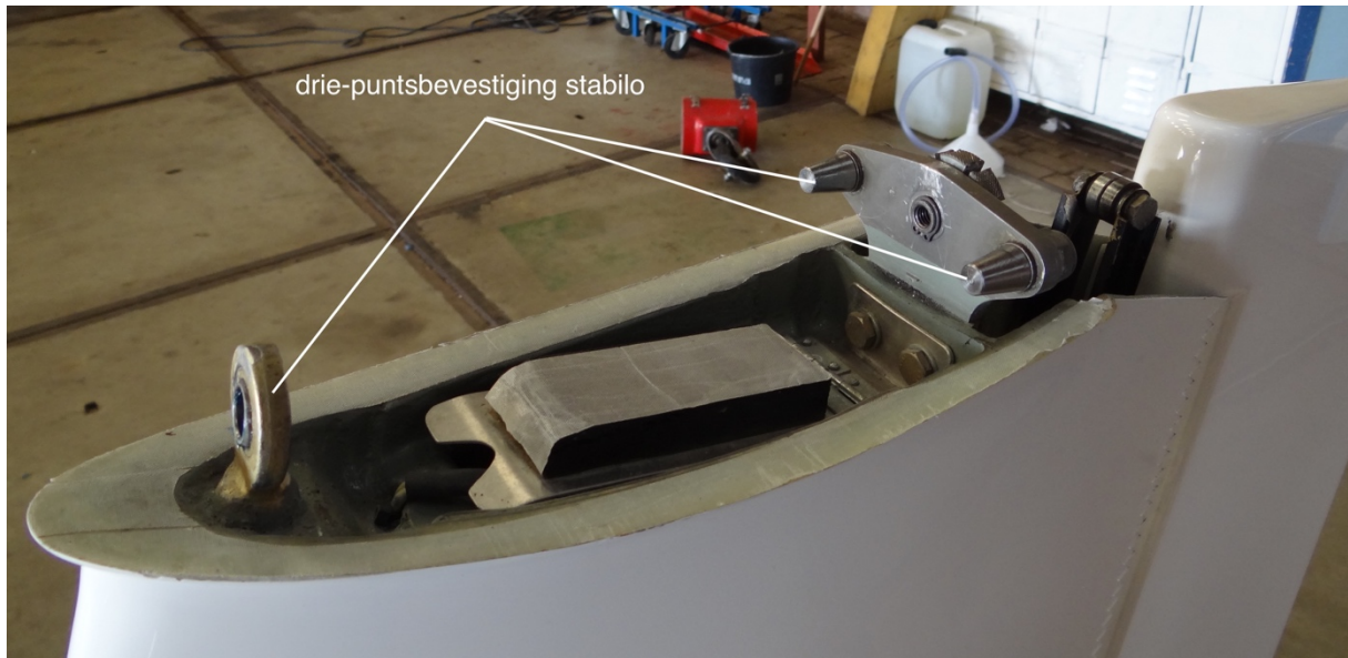
Afbeelding 1-10 Driepuntsbevestiging horizontaal stabilo (Discus-cs)
