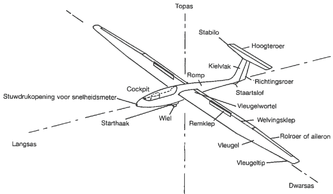
Afbeelding 1-1 Samenstellende delen
