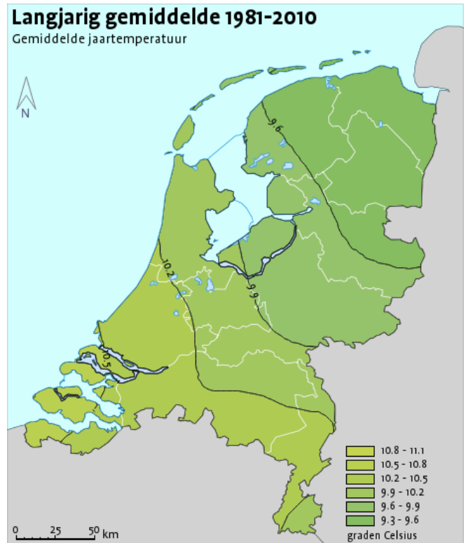
Gemiddelde temperatuur van Nederland (afb. van KNMI-klimaatatlas)
