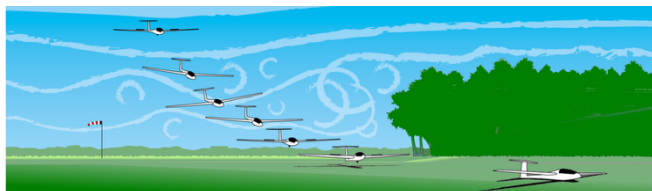
Turbulentie (voor een grotere afbeelding klik op de tekening )
