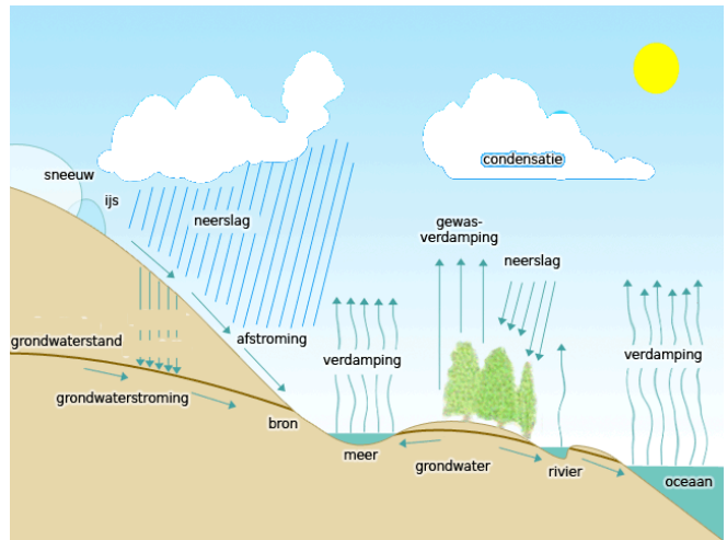
Waterkringloop (afb. van wikipedia)
